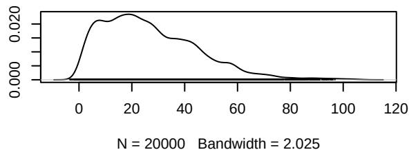
Density of d.Erlotinib.Erlotinib_ERi
