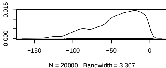
Density of d.Erlotinib.Erlotinib_Autophagyi
