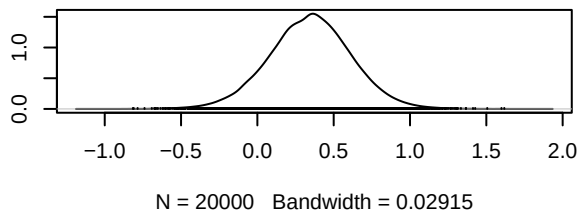
Density of d.Erlotinib.Erlotinib_antiangio
