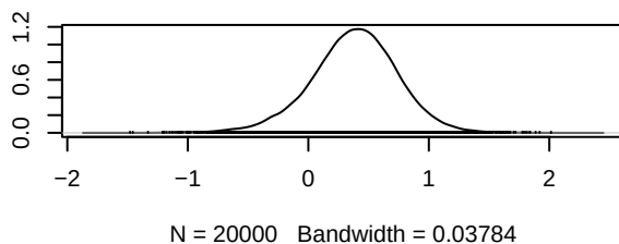
Density of d.Erlotinib.Erlotinib_METi
